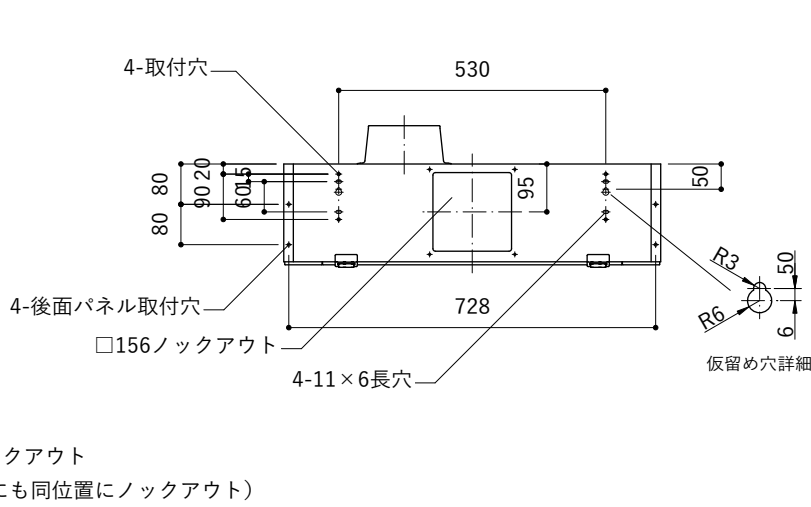
背面取付図
